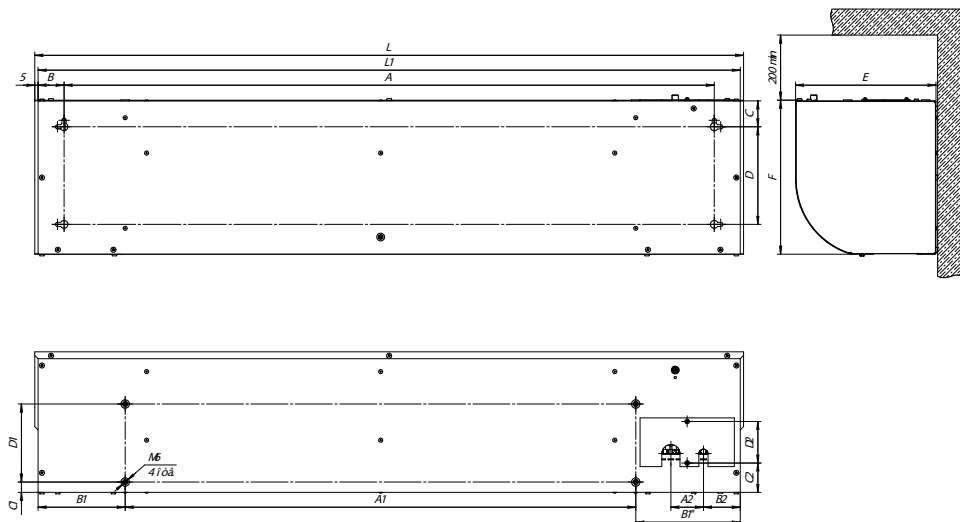
РИС. 4 Установочные размеры ZVV-1E6T 2.0, ZVV-1.5E9T 2.0, ZVV-2E12T 2.0, ZVV-2E18T 2.0, ZVV-2E24T 2.0, ZVV-9T 1м Н.
