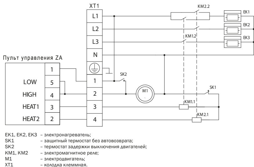
РИС. 5 Схема электрическая ZVV-1E6T 2.0, ZVV-9 1м Н, ZVV-1.5E9T, ZVV-2E12T2.0
