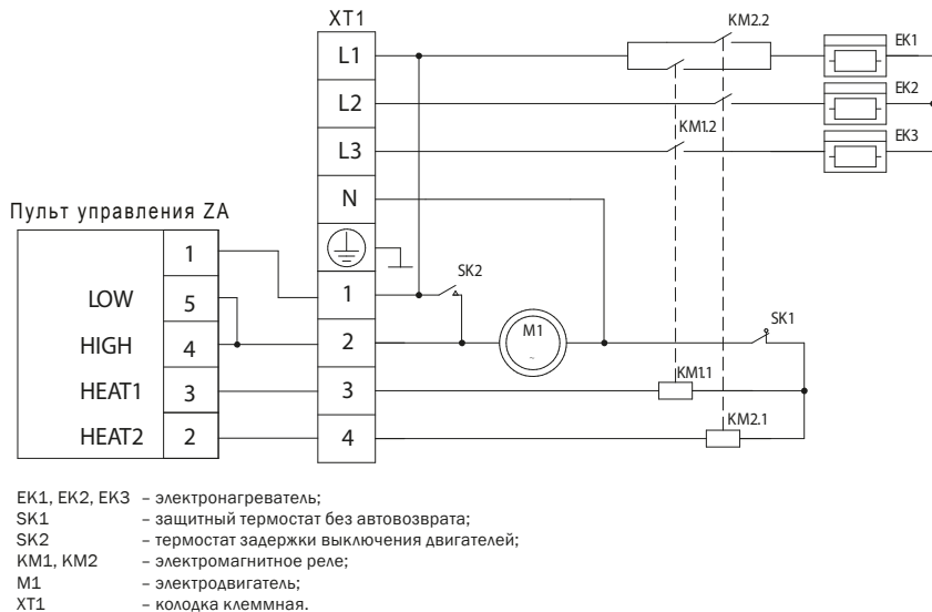
РИС. 6 Схема электрическая ZVV-2E18T 2.0, ZVV-2E24T 2.0
